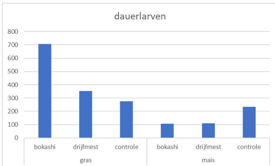
Figuur 24 Dauerlarven op grasland (bedrijf 1) en maaisland (bedrijf 2)
